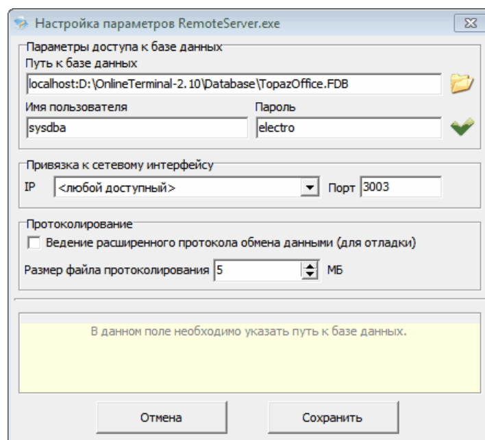
Рисунок 5. Мастер настройки "Он-лайн сервер"
