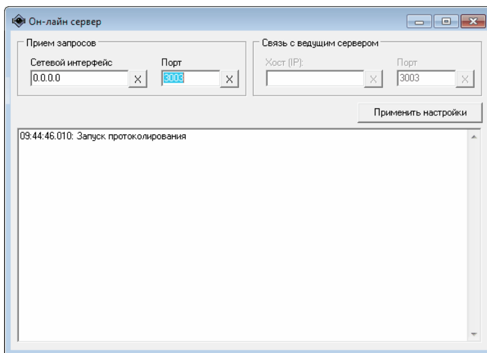
Рисунок 1. Онлайн сервер.
