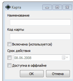
Рисунок 50. Добавление карты.
