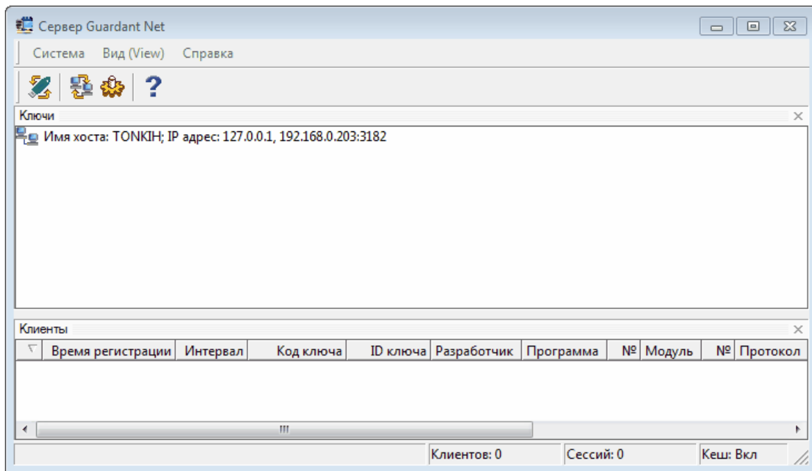
Рисунок 4. Сервер ключей.
