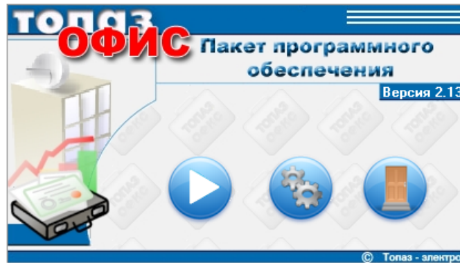
Рисунок 3. Топаз-Офис.
