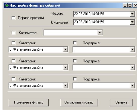
Рисунок 55. Настройки фильтра.
