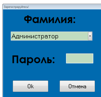
Рисунок 13. Окно регистрации
