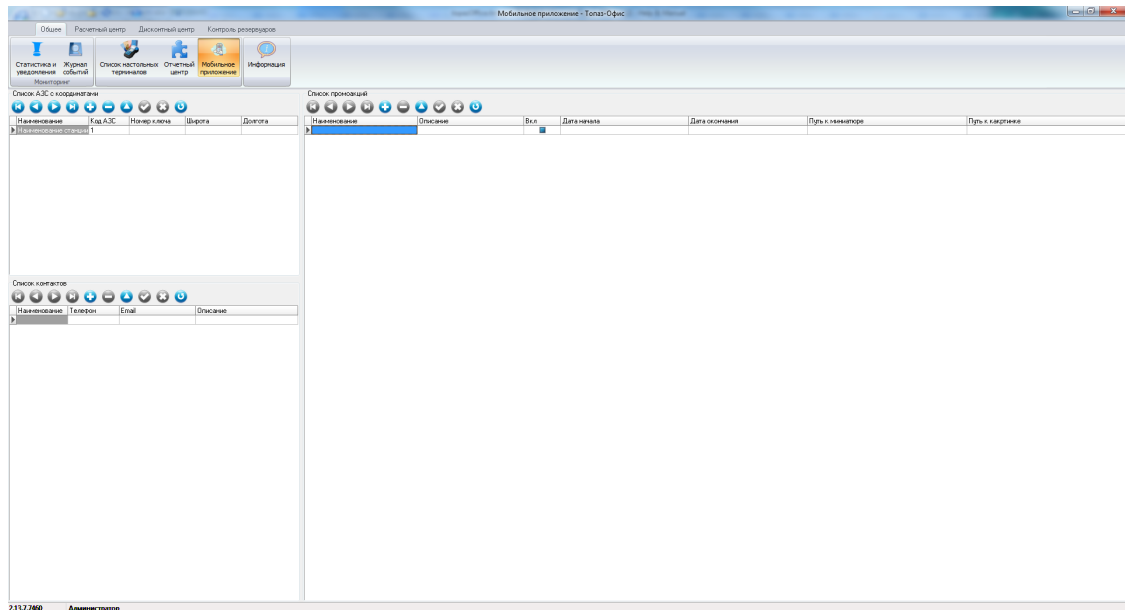
Рисунок 57. Мобильное приложение.
