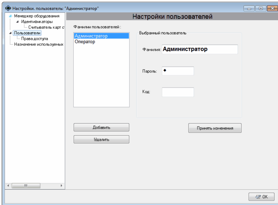
Рисунок 20. Настройки пользователей.
