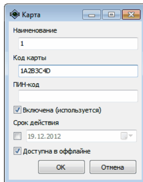
Рисунок 42. Добавление карты
