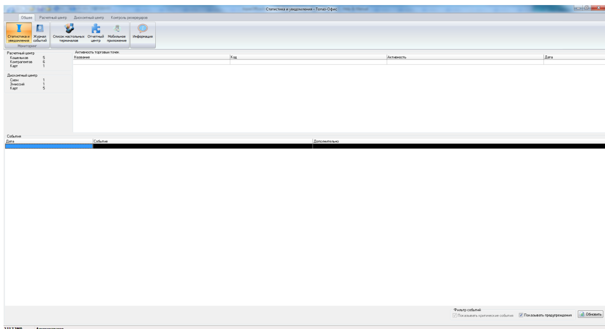
Рисунок 56. Статистика.
