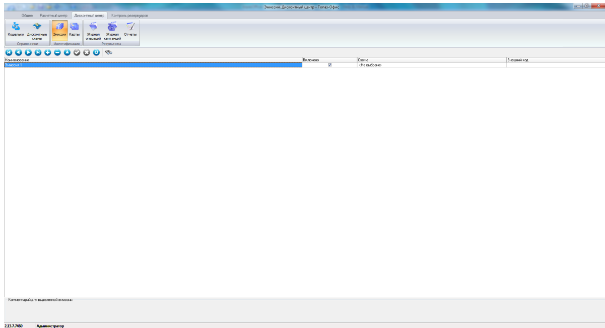
Рисунок 47. Эмиссии.
