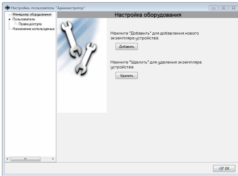
Рисунок 15. Менеджер оборудования.
