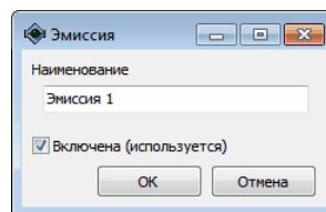
Рисунок 48. Добавление эмиссии
